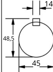
Detalhes Eixo de Saída
