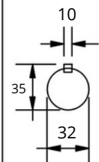
Detalhes Eixo de Entrada
