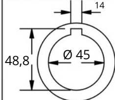
Detalhes Eixo de Saída Vazado
