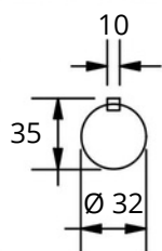
Detalhes Eixo de Entrada
