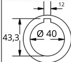
Detalhes Eixo de Saída Vazado
