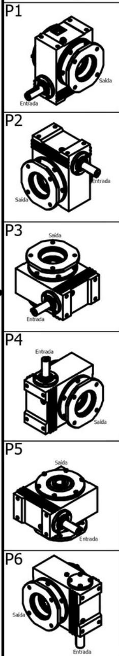
Detalhes Eixo de Entrada
