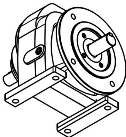
Detalhes Eixo de Entrada
