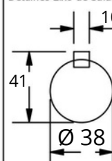
Detalhes Eixo de Saída
