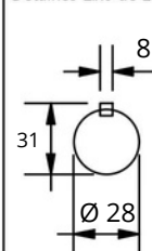
Detalhes Eixo de Entrada
