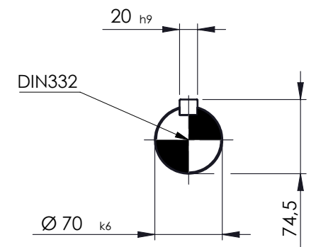
Detalhe eixo de entrada Input Shaft Detail Detalle eje de entrada (Sem escala/no scale/sin escala)
